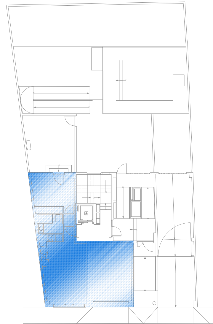
Planta Baja. E: 1/200
